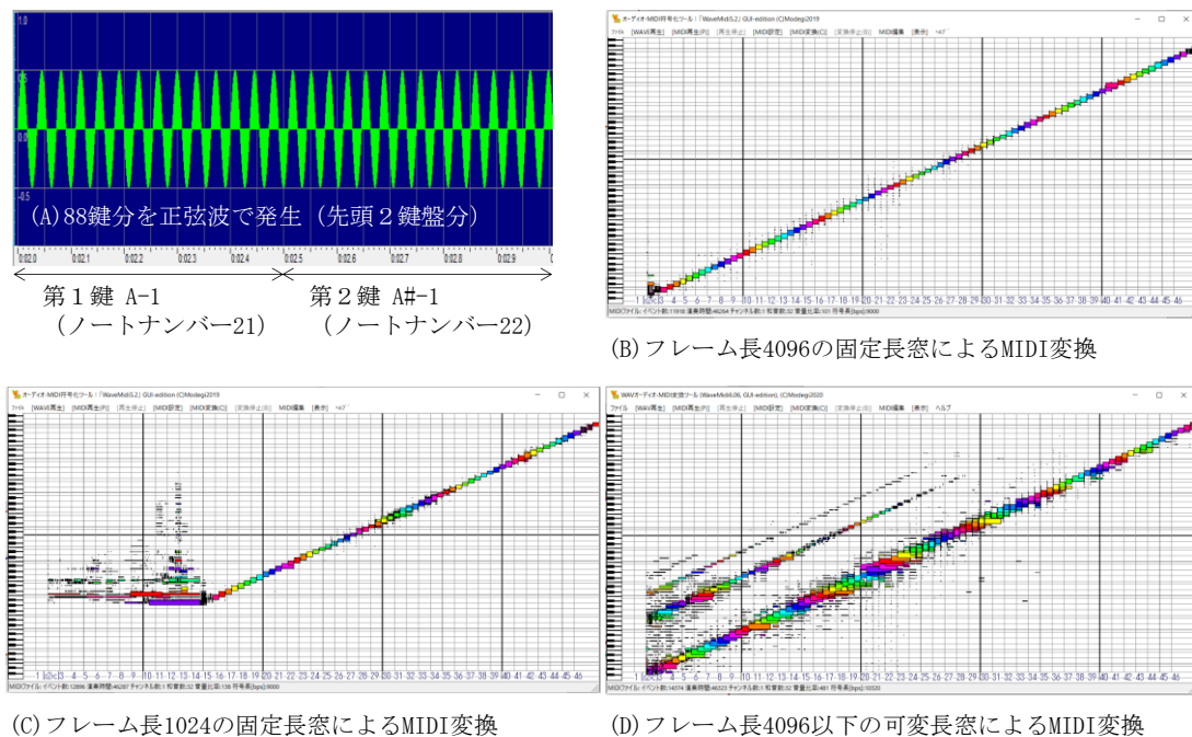
図8 ピアノ88鍵・半音階スケール（0.5秒×88）のMIDI変換例
